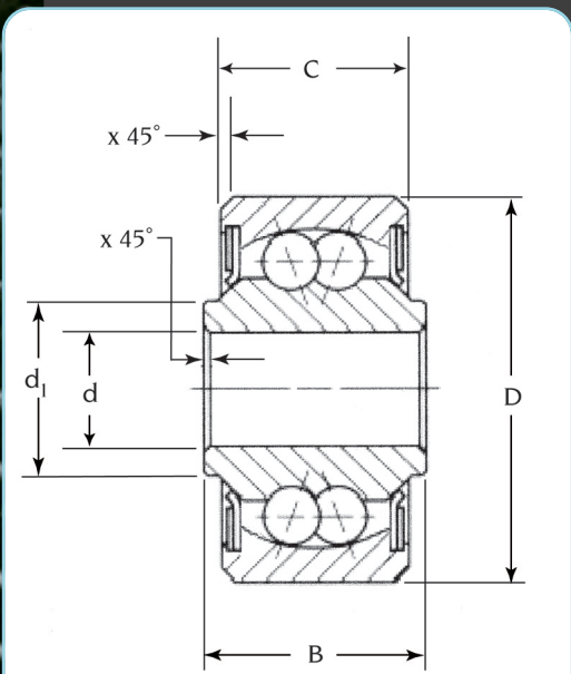
PENDELKUGELLAGER EIN- ODER DOPPELREIHIG
