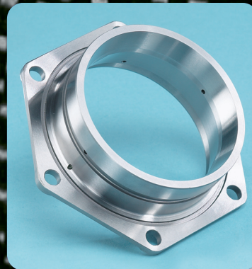
Geflanschte Doppelschale zur Aufnahme zweier Kegelrollen-Konusse, mit Ölnut und Öllöchern.
