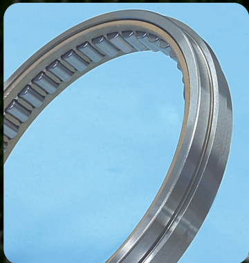
Rollenlager mit Flansch in der Mitte des Außenringdurchmessers, mit Aufnahme Nut und einteiligem Bronzekäfig.
