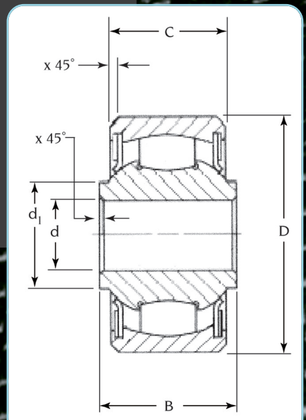
PENDELROLLENLAGER EIN- ODER DOPPELREIHIG
